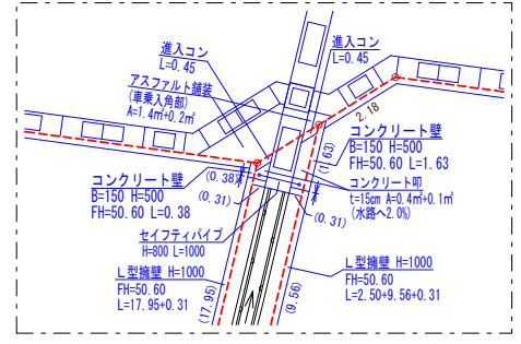
部分拡大図 1/200
