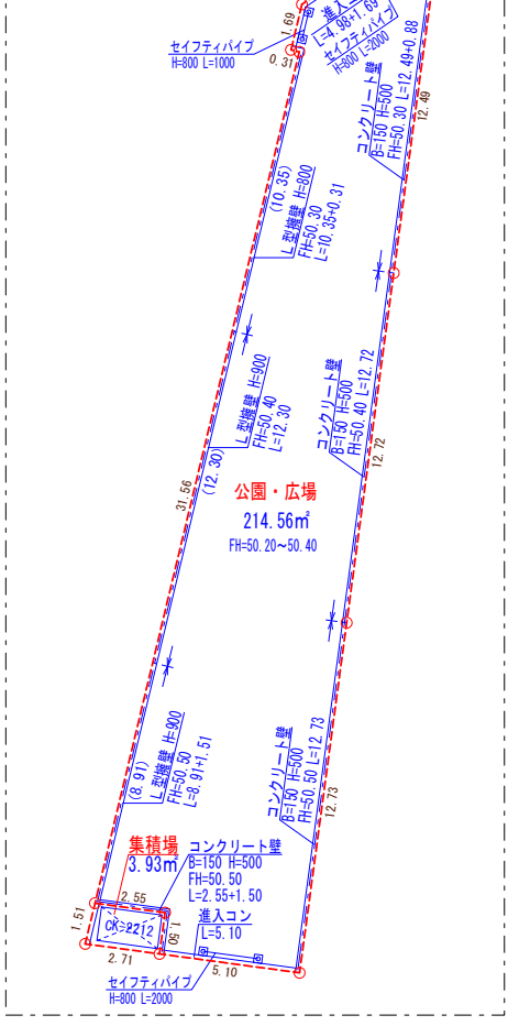
公園・広場・集積場 部分拡大図 S=1/300
